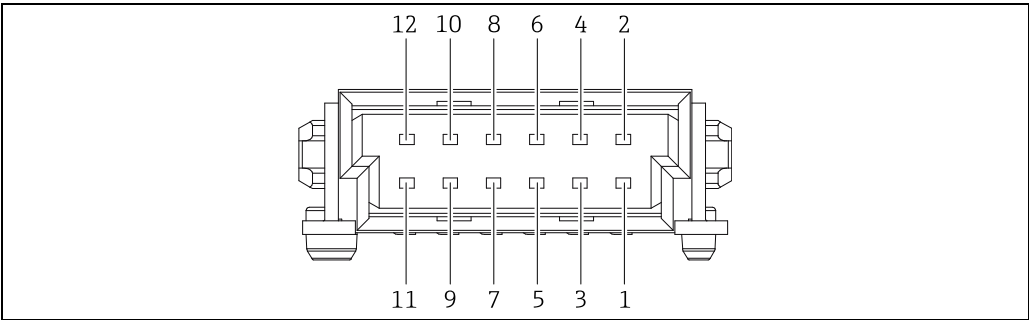
Pin-Belegung_Anschlussstecker
