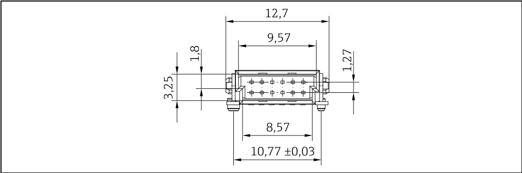
Maße_Anschlussstecker
